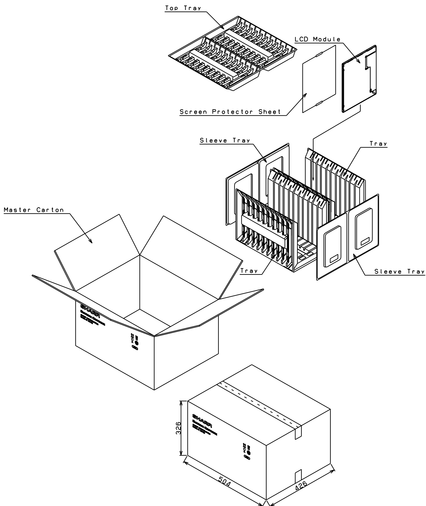
図3. 包装形態図
